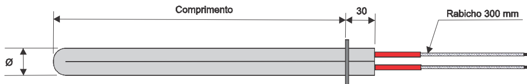
Saída com arruela de encosto
