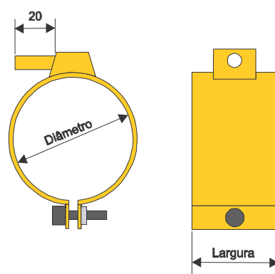
Saída 180° - Tangencial 90°
