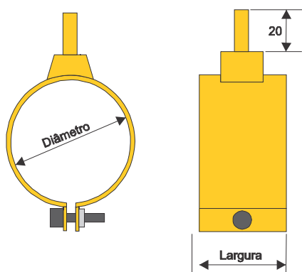
Saída 180° - Reta
