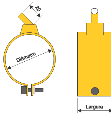
Saída 180° - Tangencial 45°
