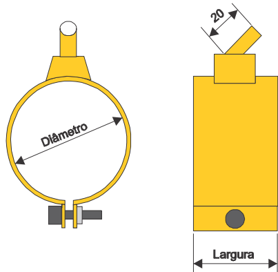
Saída 180° - Axial 45°
